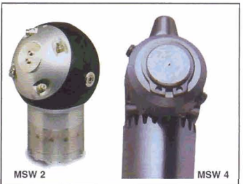
MSW 2 - MSW 4 HYDRAULIC ROTATING HEAD TÊTE HYDRAULIQUE TOURNANTE CABEZA ROTATORIA HIDRÁULICA TESTA ROTANTE ELETTRICA IDRAULICA
