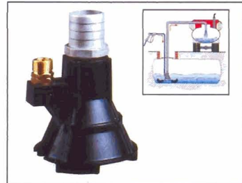
SAM 56 VACUUM CLEANER ASPIRATEUR LIQUIDES ASPIRADOR DE LIQUIDOS ASPIRATORE LIQUIDI
