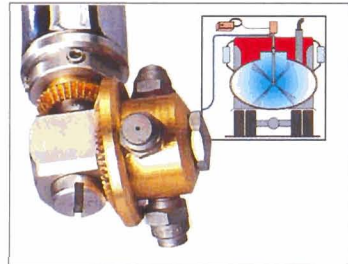
MSW 3 ELECTRIC ROTATING HEAD TÊTE ELECTRIQUE TOURNANTE CABEZA ROTATORIA ELECTRICA TESTA ROTANTE ELETTRICA
